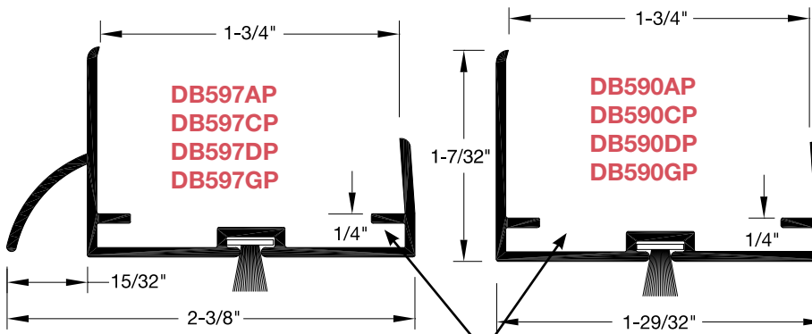
Door Extenders
